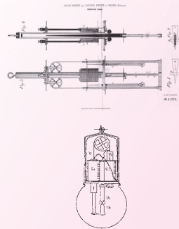
1880 OBLOUKOVÁ LAMPA
