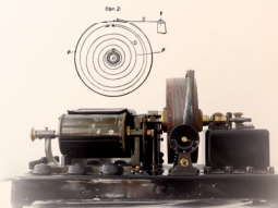
1959 POLAROGRF
